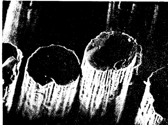
THORNEL 300 GRADE WYP 90 2 μm
