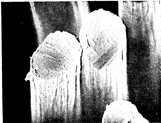
THORNEL 300 GRADE WYP 30 2 μm
