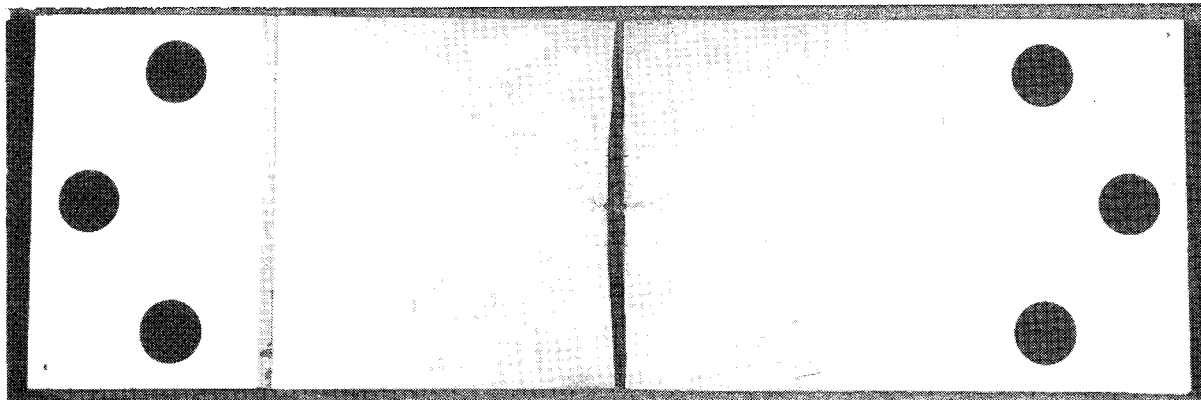
a. BONDED SKIN
