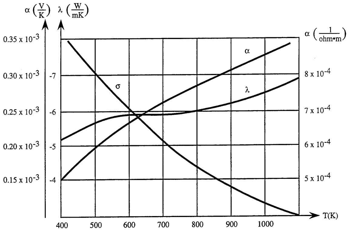
a) N-type SiGe
