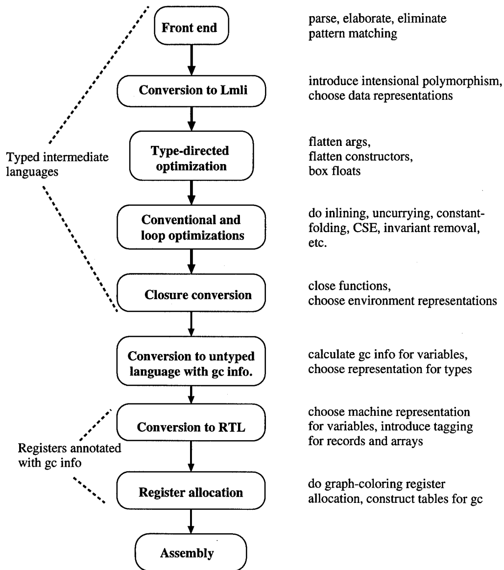
Figure 1: Phases of the TIL compiler
