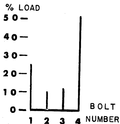
(d) Specimen 4
