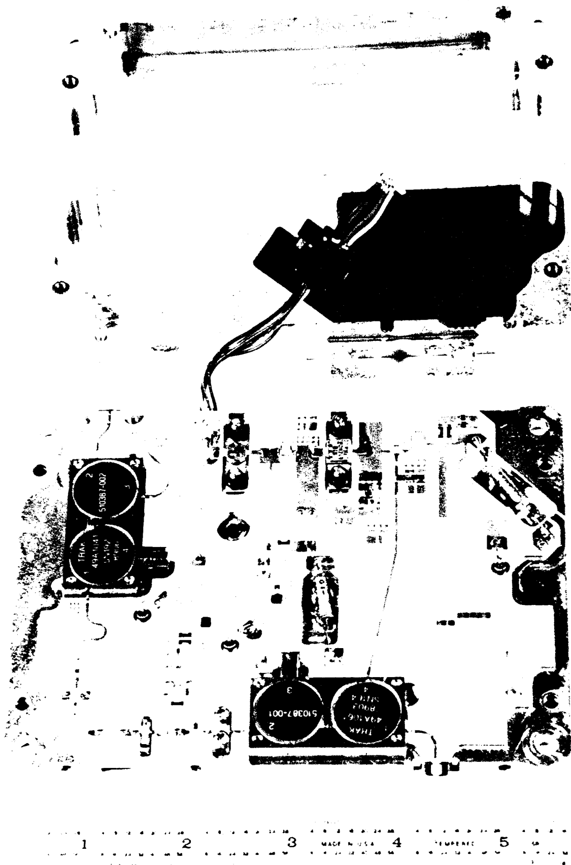
Figure 7-7. SIR-C L-band T/R module.
