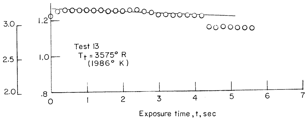
(d) Large-grain material tested in nitrogen.
