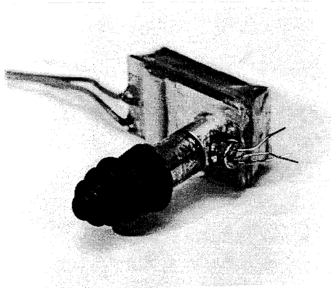
Fig. 10 Telefoon en microfoon samengebouwd met een Racal oordop.
