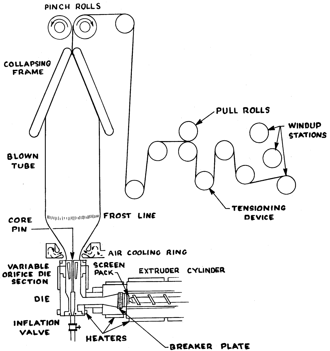
UTG FILM EXTRUDER SCHEMATIC
