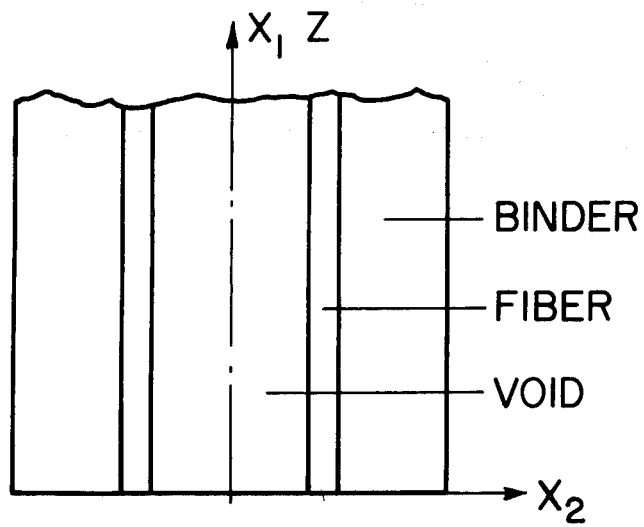
a.) SECTION
