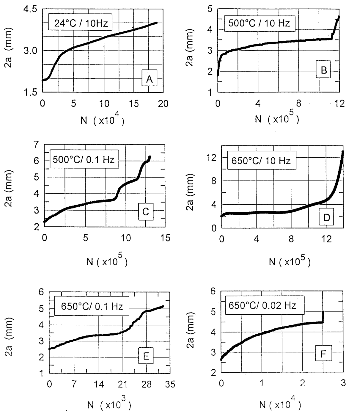
Fig. 5.3 Variation of the crack length, 2a , with the number of fatigue cycles, N , for different test conditions. (a) 24^{\circ}\text{C} / 10\text{Hz} ; (b) 500^{\circ}\text{C} / 10\text{Hz} ; (c) 500^{\circ}\text{C} / 0.1\text{Hz} ; (d) 650^{\circ}\text{C} / 10\text{Hz} ; (e) 650^{\circ}\text{C} / 0.1\text{Hz} ; (f) 650^{\circ}\text{C} / 0.02\text{Hz} .
