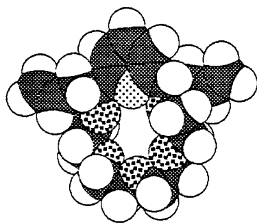
( S,S )-4a
