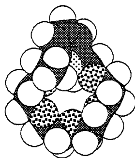
( S,S )-5a
