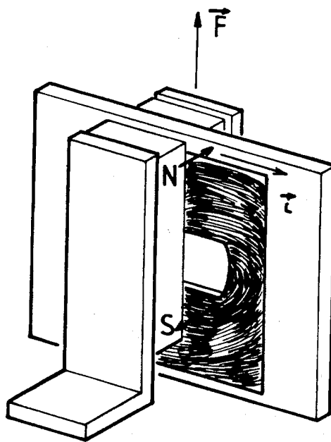
Fig. 3 Actuator principle
