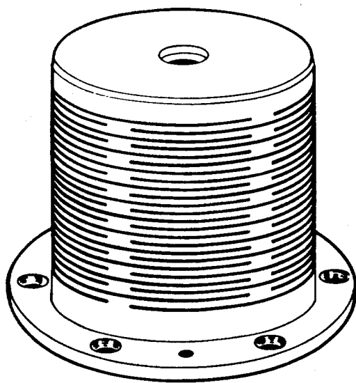
Fig. 2 Flexible pivot
