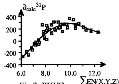
Fig.3: \text{PXYZ}
