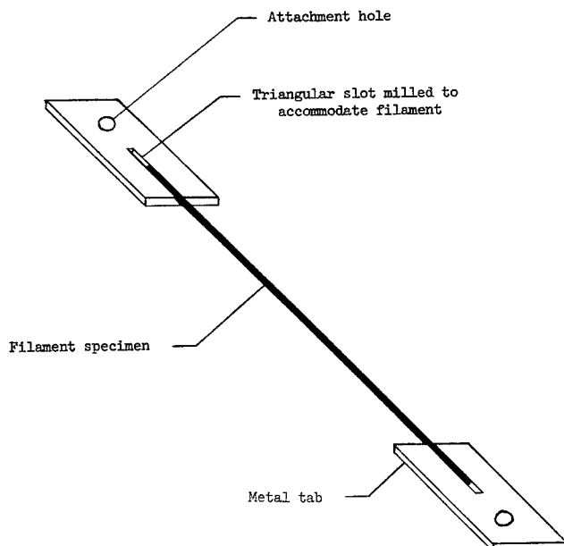
Figure 2.- Filament tensile specimen.
