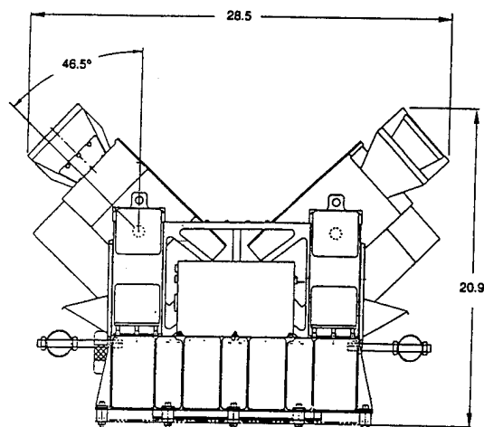
Fig. 7 The MAXIE instrument.
