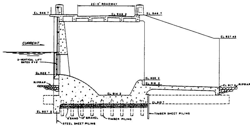
SECTION D-D
