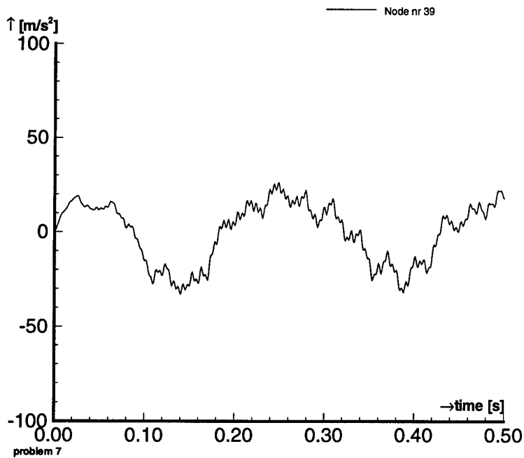
fig. A.7.10 Versnelling som 7 vloer n.p. 39.
