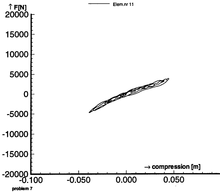
fig. A.7.24 Veer karakteristiek som 7 element 11.
