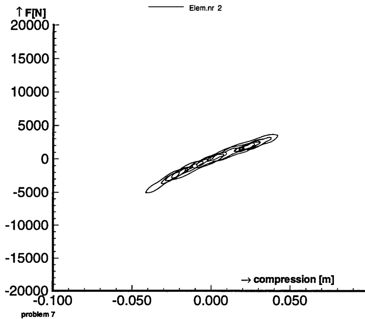
fig. A.7.21 Veer karakteristiek som 7 element 2.
