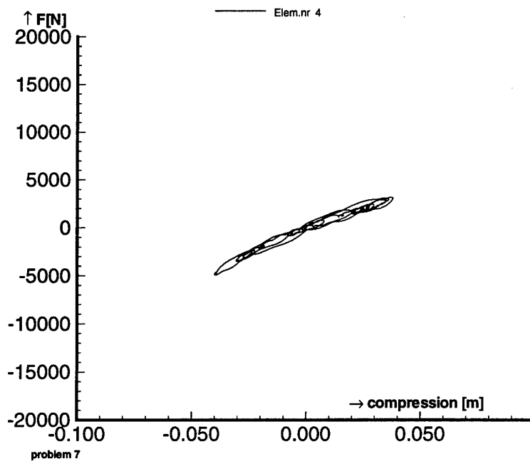
fig. A.7.22 Veer karakteristiek som 7 element 4.
