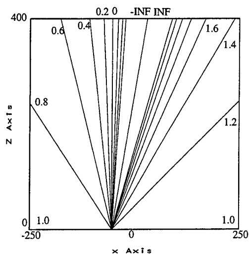
(d) x_0 = -50, x_{0e} = 0, \beta_f = 0.2
