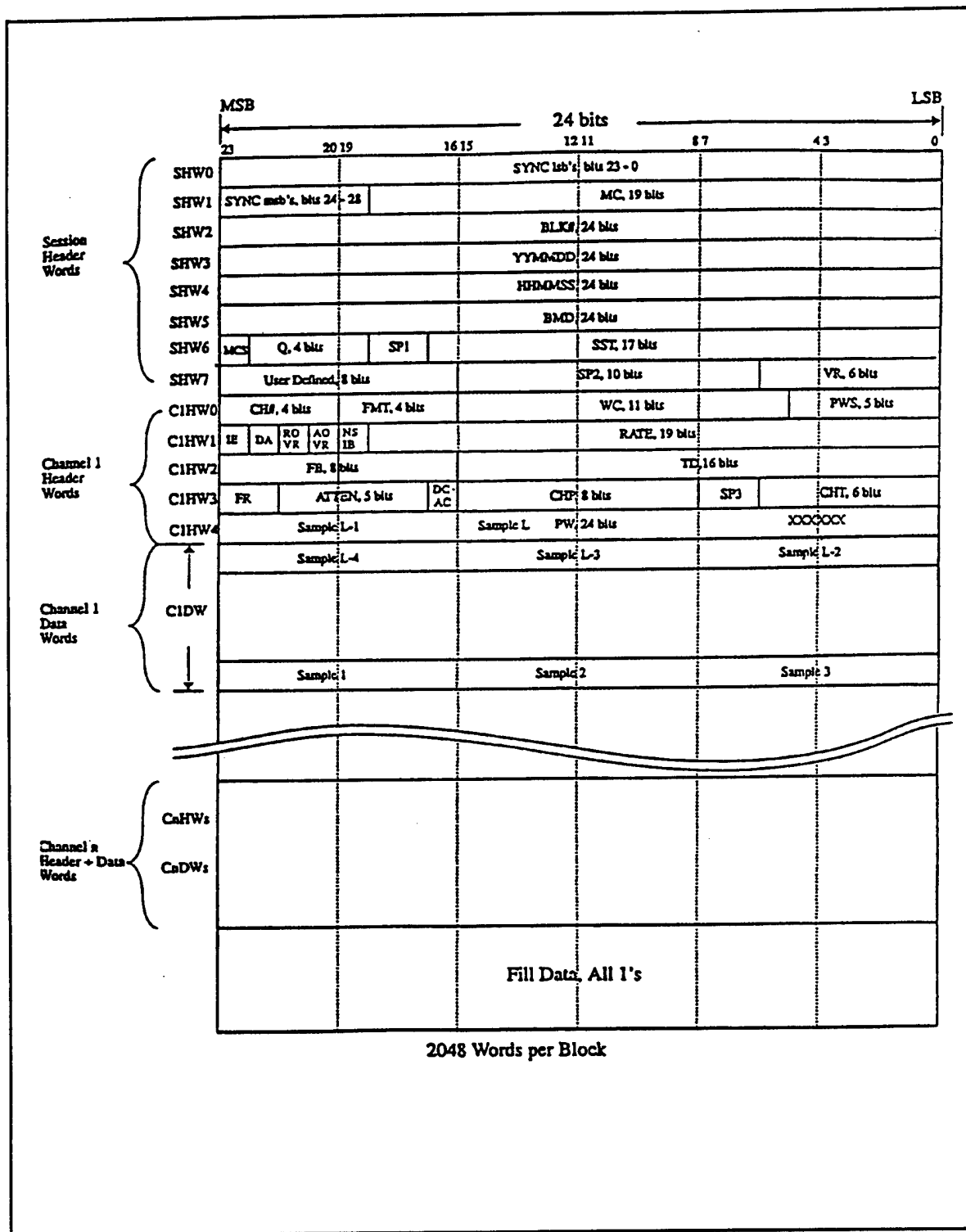
Figure 6-8. ADARIO data format.
