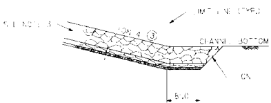
RIPRAP TRENCHFILL 3
