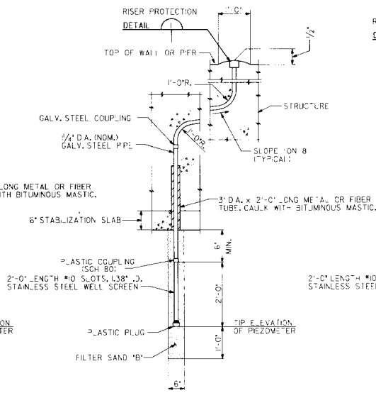
TYPE B PIEZOMETER
