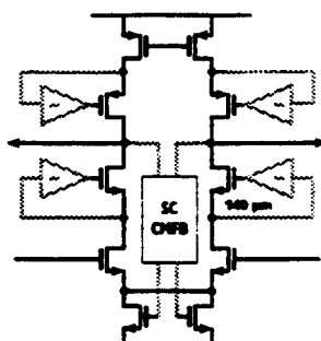
Fig.3. Super cascode op amp circuit.
