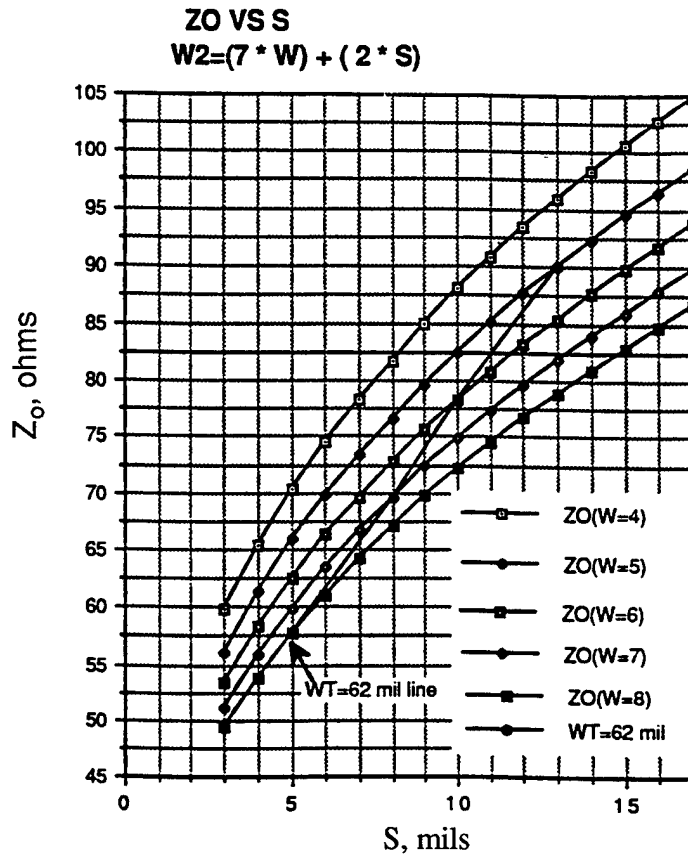
FIGURE 4. Coplanar Waveguide ( T = 25 , ER = 10 ).
