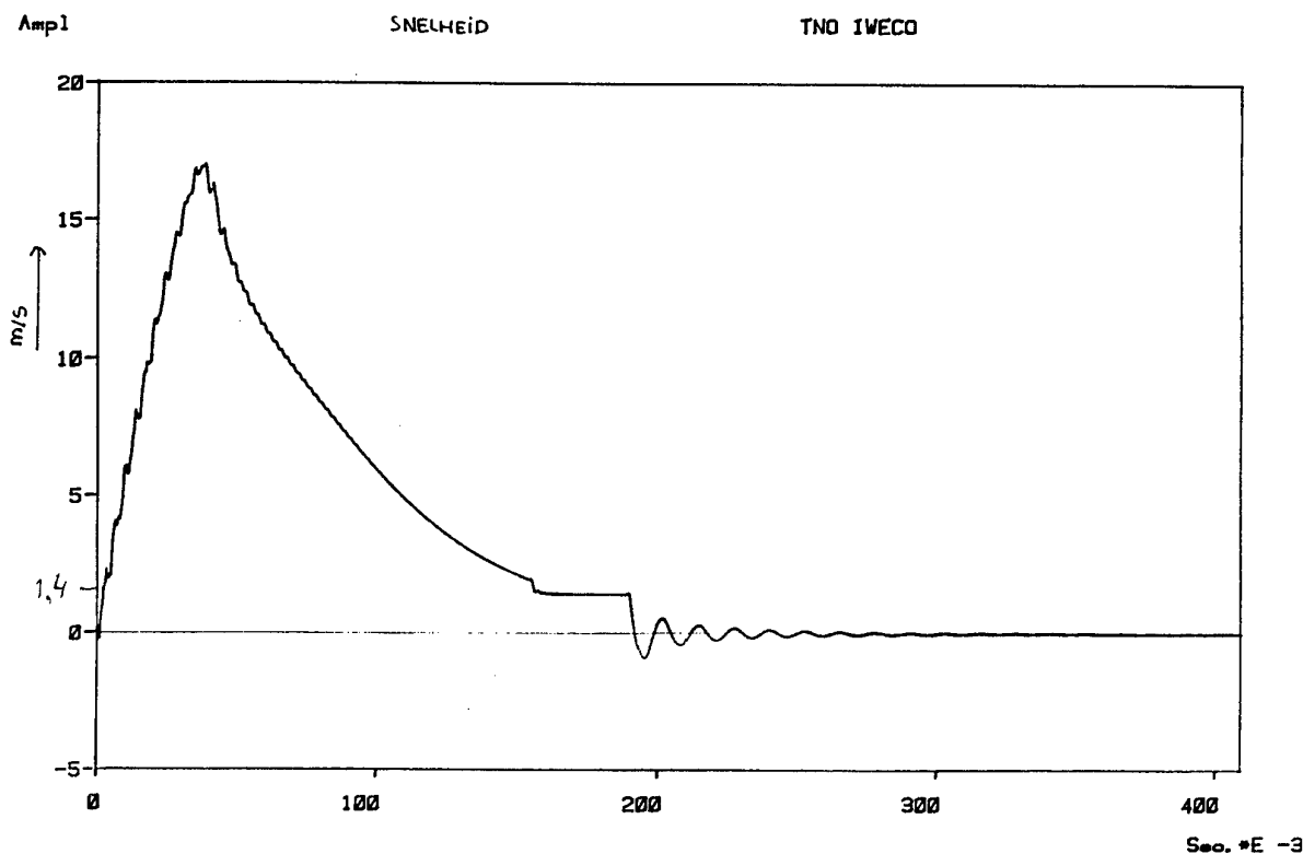
Fig 6. Gesimuleerde verplaatsing en snelheid. Uitgangspunt: 1,2 meter opspanlengte. Bijzonderheid: snelheidssprong van 1,4 m/s 2 na 200 ms.
