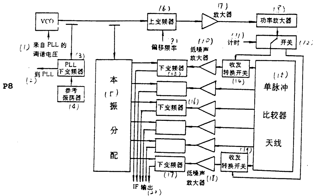
图9 多功能毫米波射频前端
