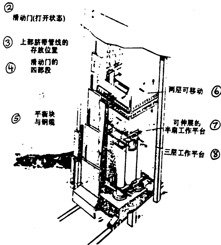
① 图 2 最后组装厂房里面的三层工作平台
