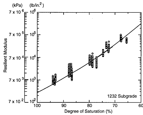
b. 1232 subgrade.
