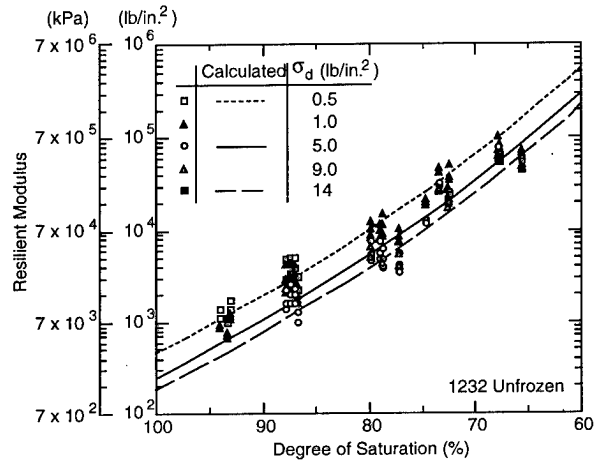
b. 1232 subgrade.
