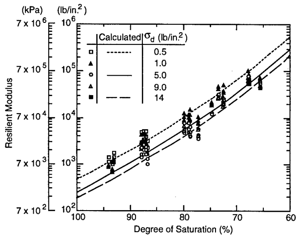
b. 1232 subgrade.
