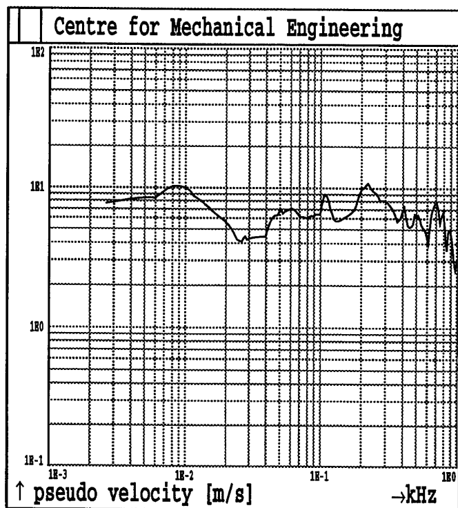
Fig.2B85. Shot 2 MAXIMAX Sensor A5
