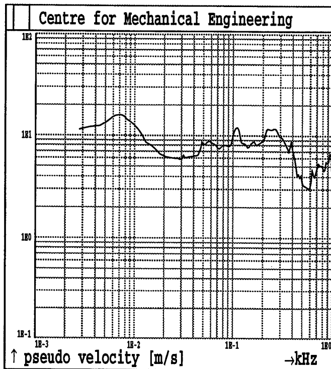
Fig.3B85. Shot 3 MAXIMAX Sensor A5
