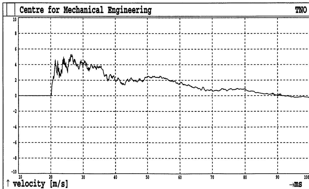
Fig.2B34. Shot 2 Sensor A2
