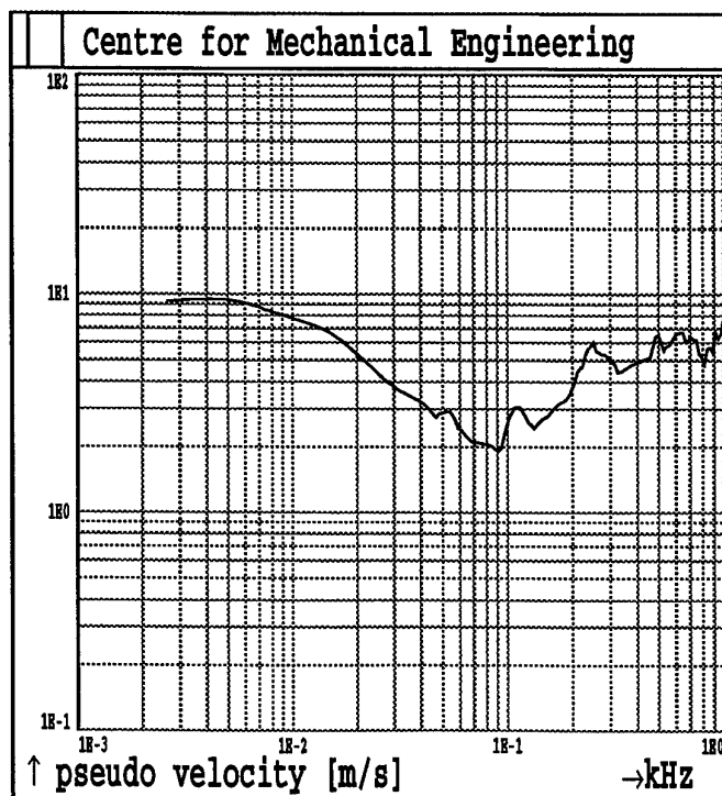
Fig.2B84. Shot 2 MAXIMAX Sensor A4
