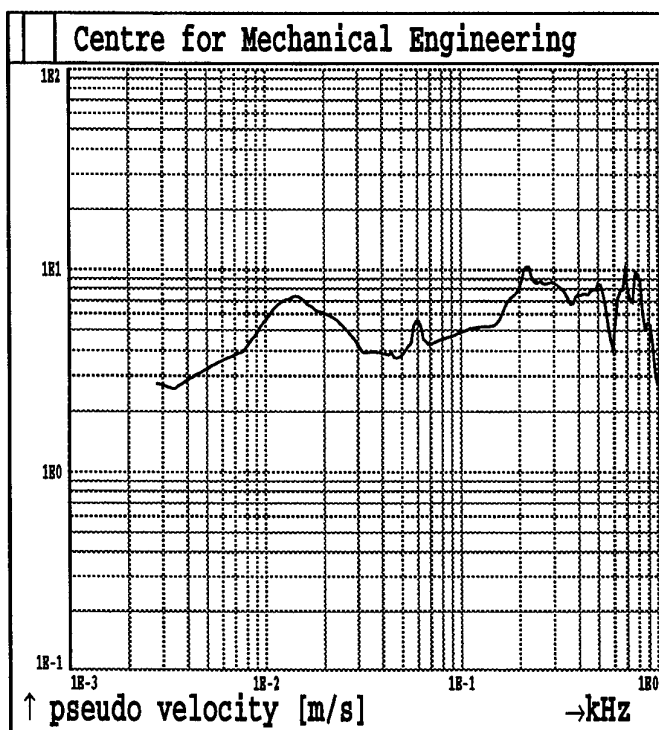
Fig.1B85. Shot 1 MAXIMAX Sensor A5
