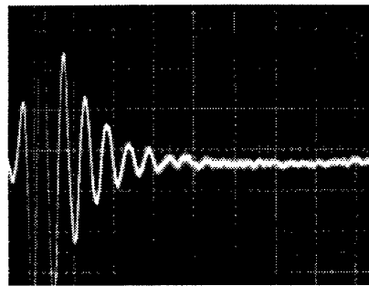
Fig. 4.7.2.1b 4 GHz
