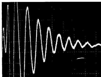
Fig. 4.7.2.1c 2 GHz
