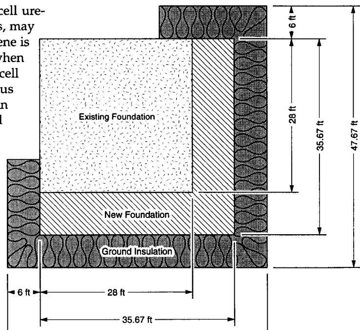
a. Foundation plan.
