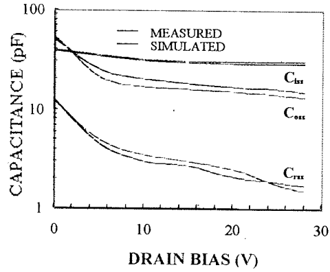
Fig.4 C-V Plots
