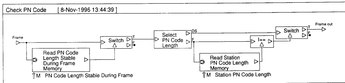
Figure A-10. Check PN Code Simulation Module
