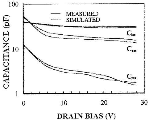
Fig.4 C-V Plots
