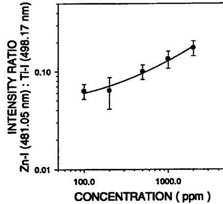
(d) Kaolin
