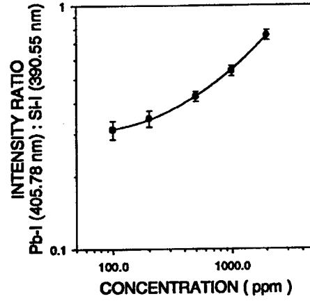
(b) Silt
