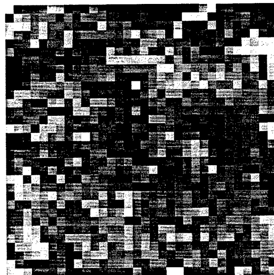
(d) GLCM
