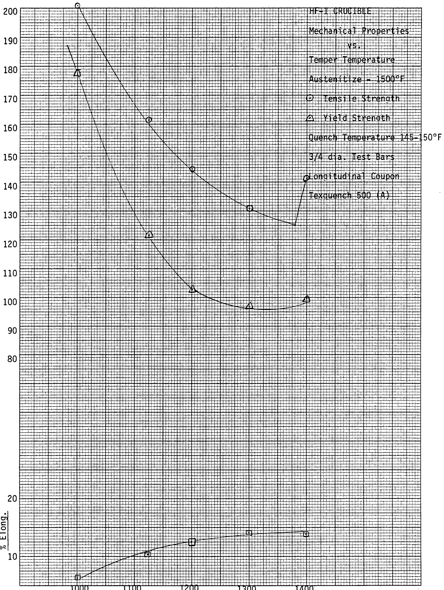
Fig. 12 Tempering Temperature (°F)
