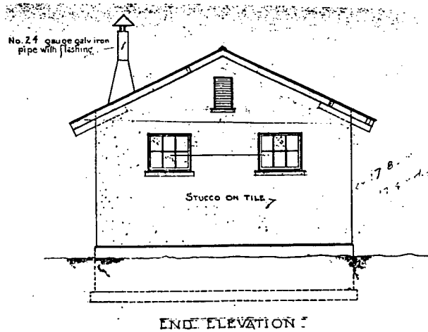
END ELEVATION
