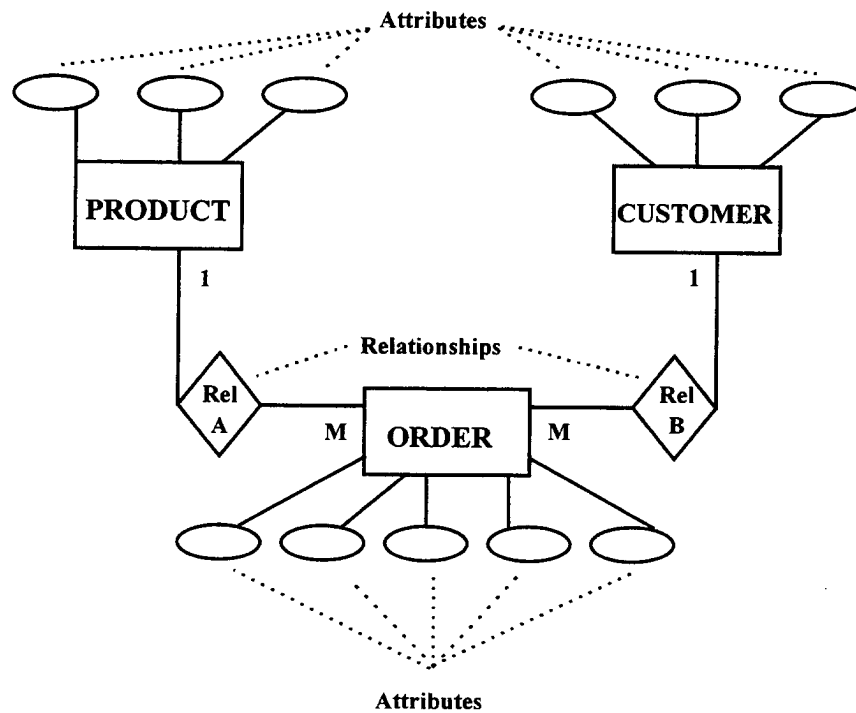
Figure 8. The ER Diagram
