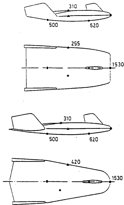
Fig 12 Maximum surface temperatures (°C)
