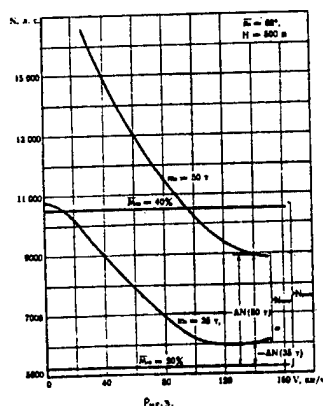
Рис. 3. Зависимость потребляемой и располагаемой мощности от скорости полета вертолета Ми-26.
