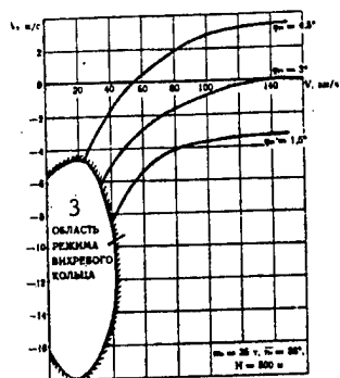
Рис. 2. Зависимость вертикальной скорости снижения от скорости планирования вертолета Ми-26.
