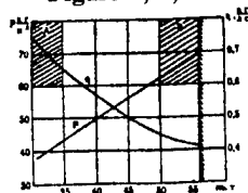
Рис. 1. Зависимость нагрузки на обметаемую несущим винтом площадь и энерговооруженности от полетной массы вертолета Ми-26.
