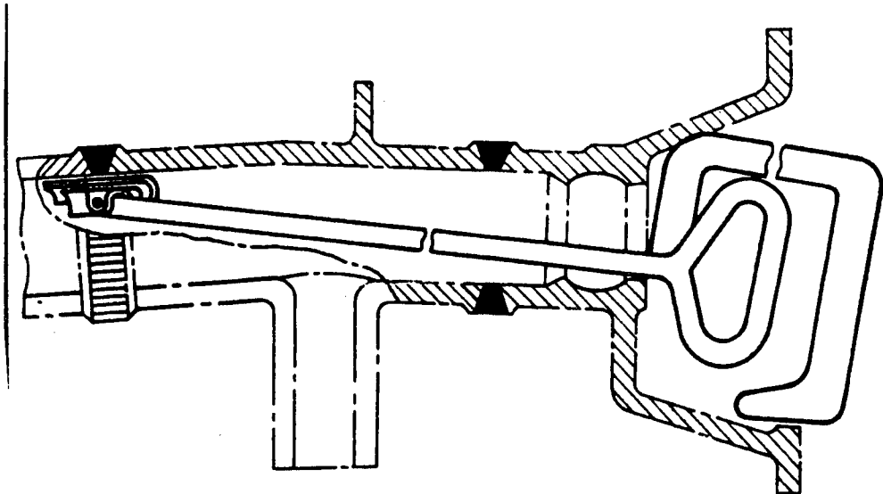
Устройство для рентгеноконтроля швов сварных соединений.
