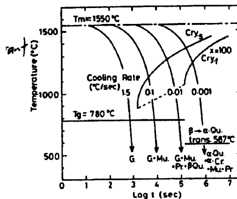
Cry : Crystallization, S : start, f : finish, X : Crystallinity (%), trans.: transformation, Mu.: Mullite, Pr. : Protoenstatite, G : Glass, Qu: Quartz.
