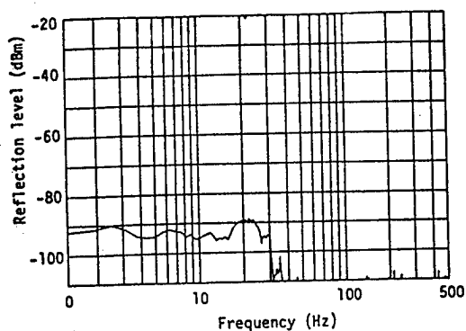
(a) 取付け台の反射レベル
