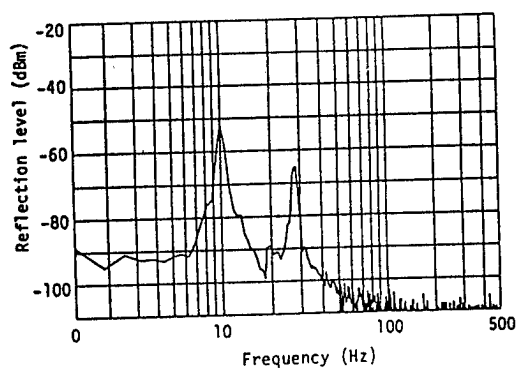
(f) R_1 = 110 cm の場合
