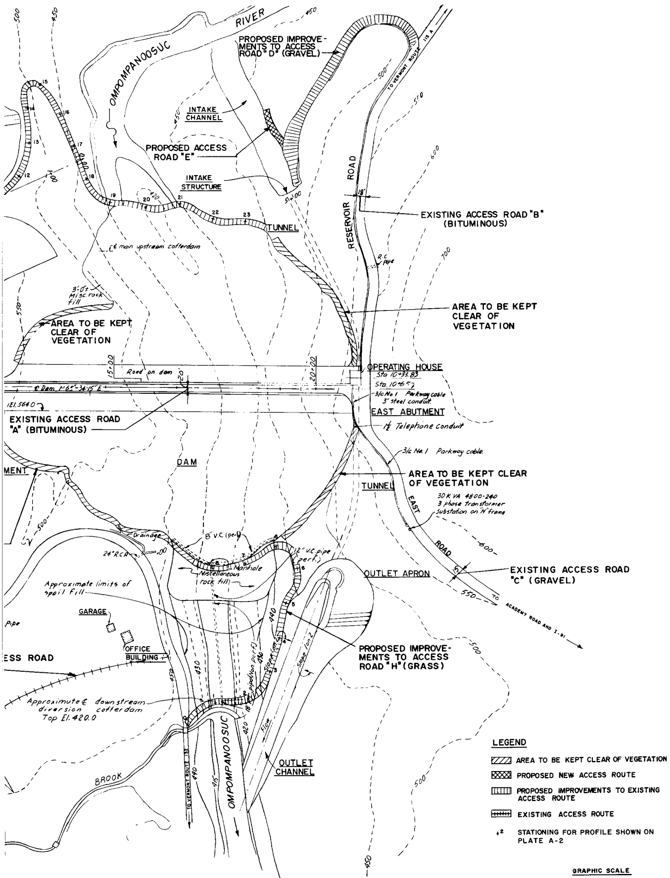
PLAN SCALE: 1"=100'
