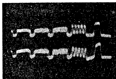
图6 视频信号：原始信号(上)，译码后信号(下)
