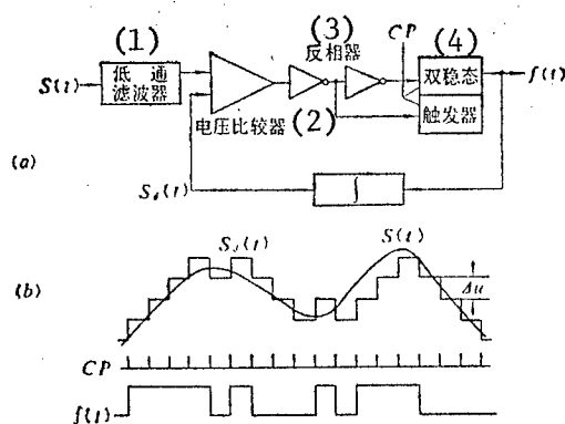
图5 增量调制方框图及波形图
