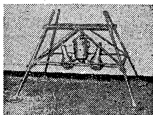
图6 固定型摄像机装置
