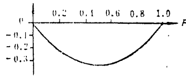
Nonlinearity (% F.S.)
