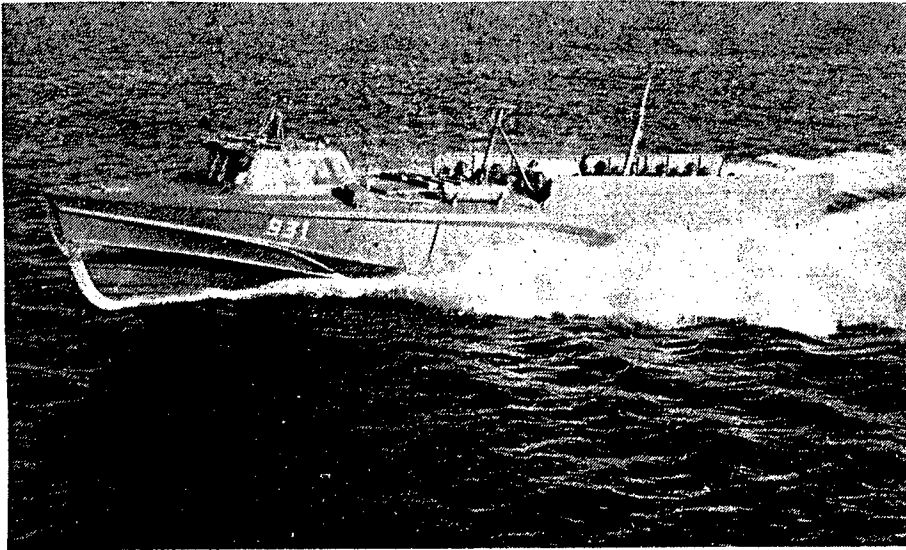
LTS-Boot Projekt „68 200“ in Transportvariante
