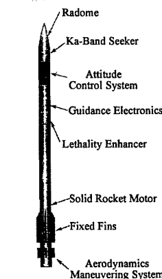
PATRIOT (PAC-3)
