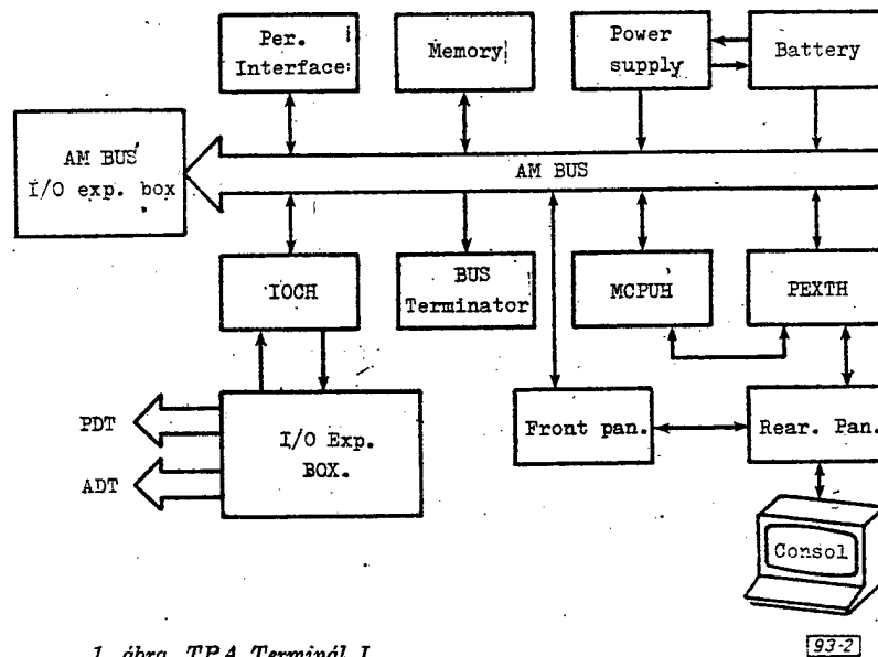
1. ábra. TPA Terminál I.
