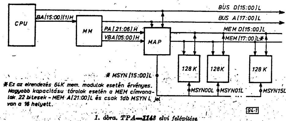
1. ábra. TPA-1148 elvi felépítése
