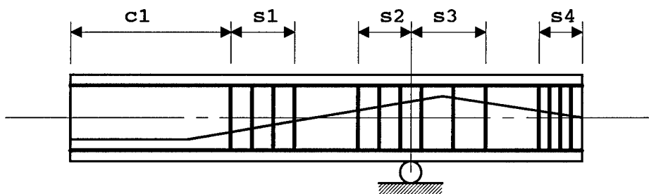
(b) Stirrups
